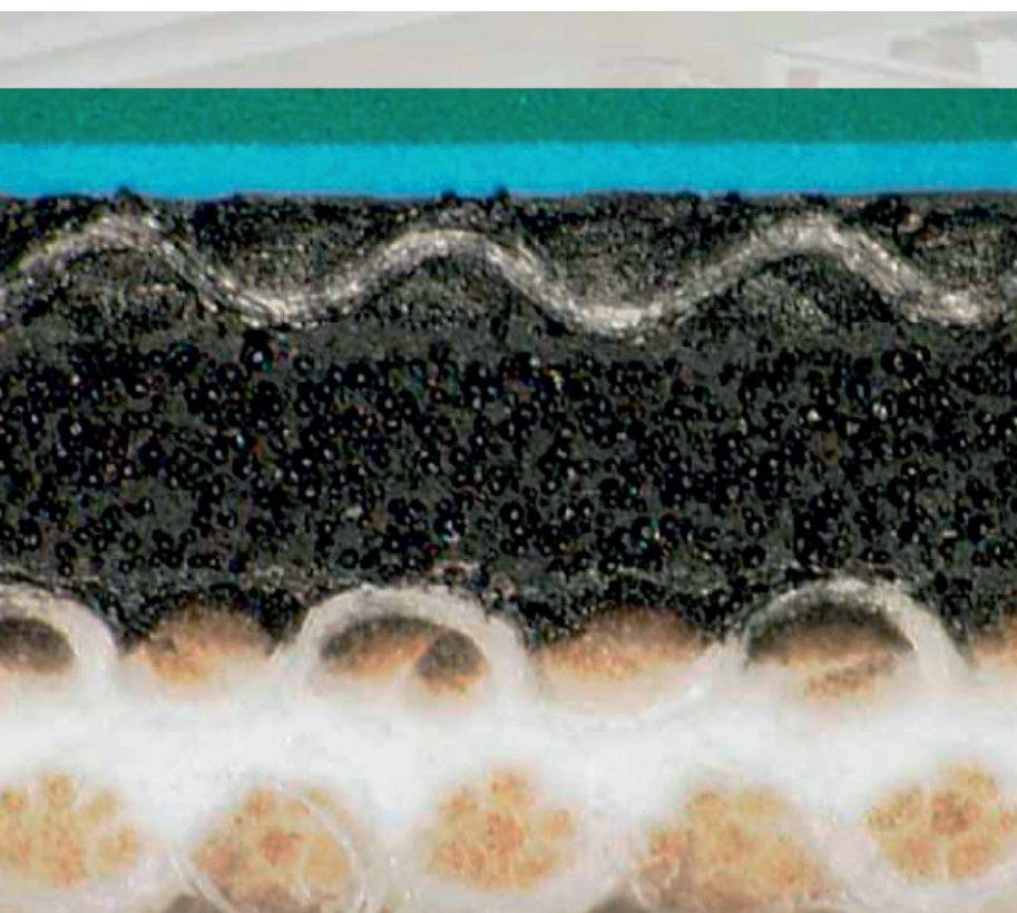
Průřez ofsetovým potahem Perfect Dot DURO
